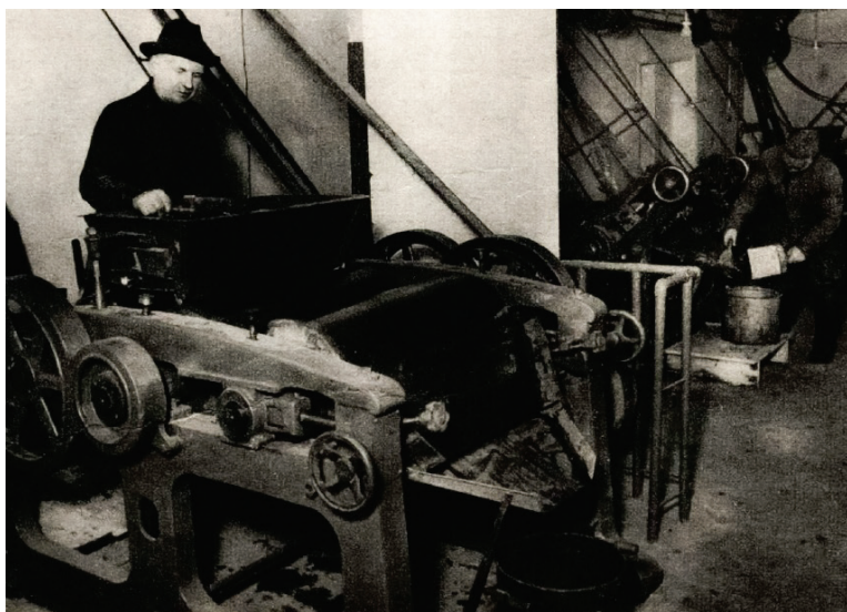
Eļļas krāsas malšana. Meistars Kārlis Krastiņš, 1941.g.
